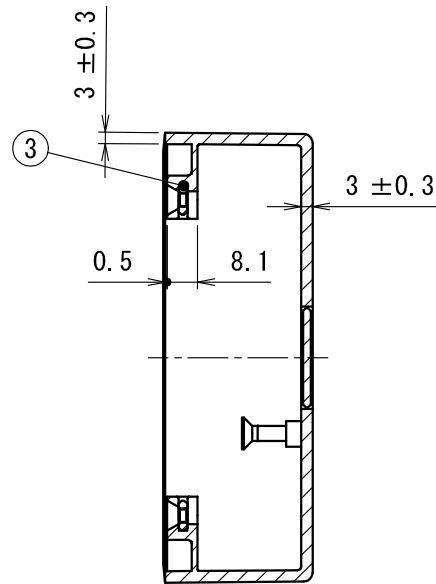
断面 A-A
